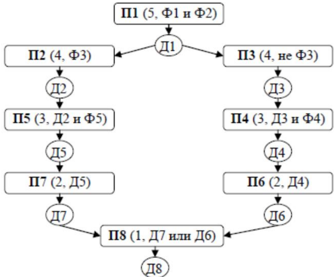
Рис. 2. Схема продукций предметной области «Ресторан».
