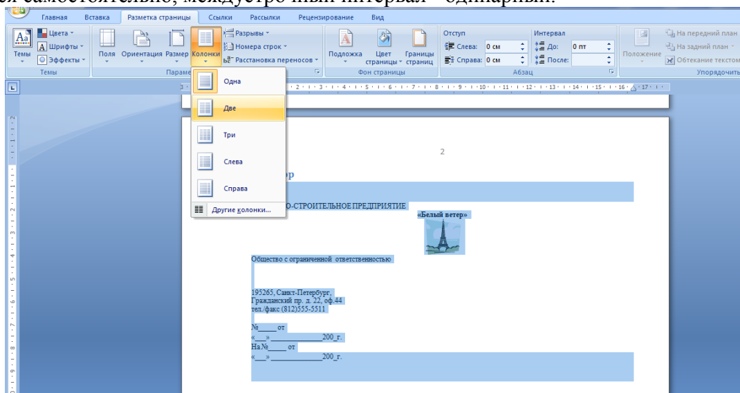
Рисунок 3. Оформление колонок
