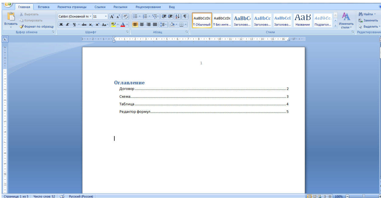
Рисунок 17. Оглавление
