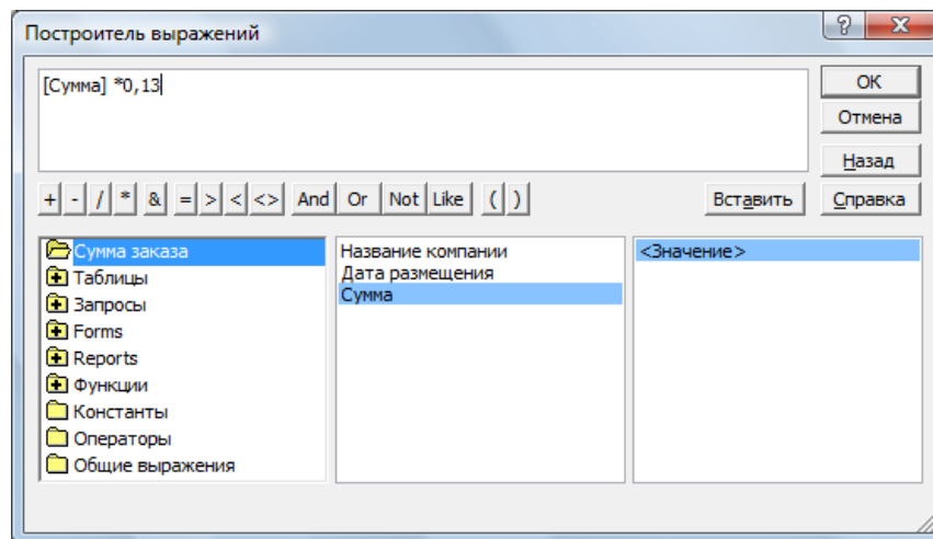
Рис. 8. Построитель выражений
