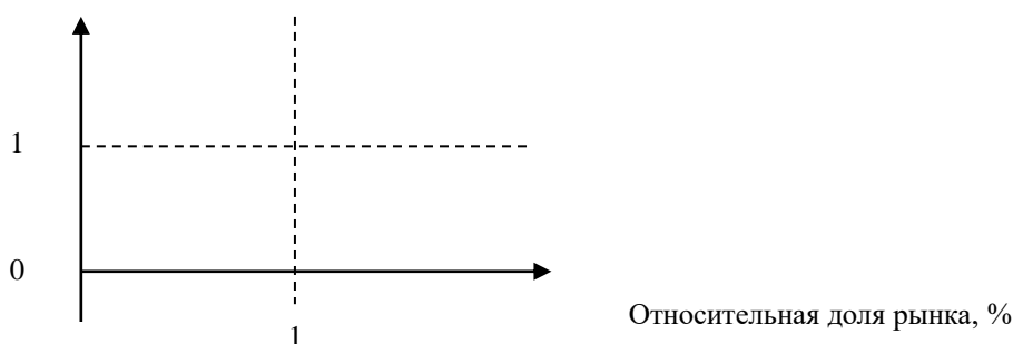
Рисунок 1 – Матрица БКГ
