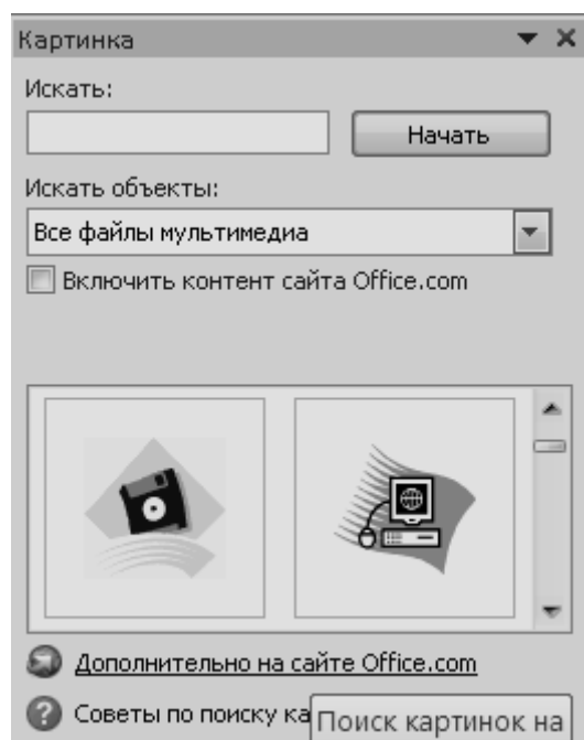
Рисунок 5 – Вставка картинки
