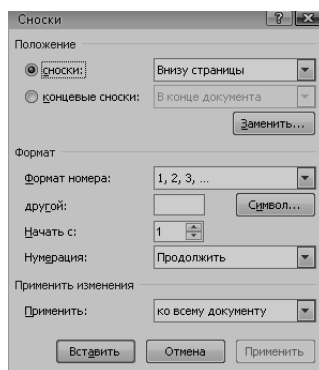
Рисунок 2 – Вставка сносок
