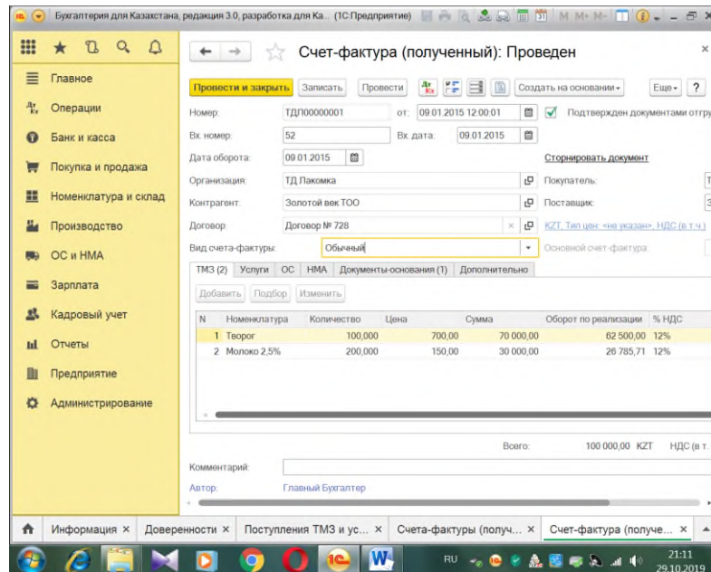
Рисунок 12 – Счет-фактура
