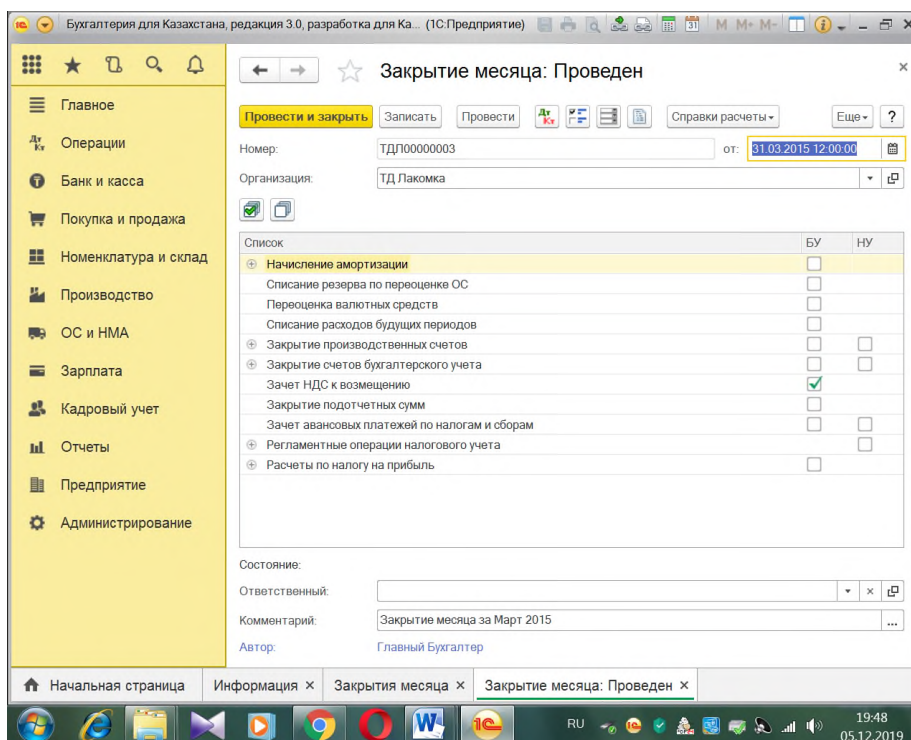
Рисунок 23 – Заккрытие месяца
