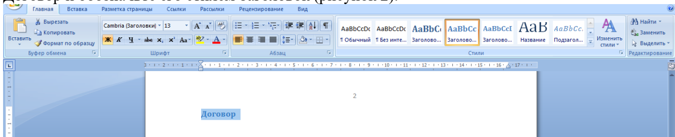
Рисунок 2. Оформление стилей
