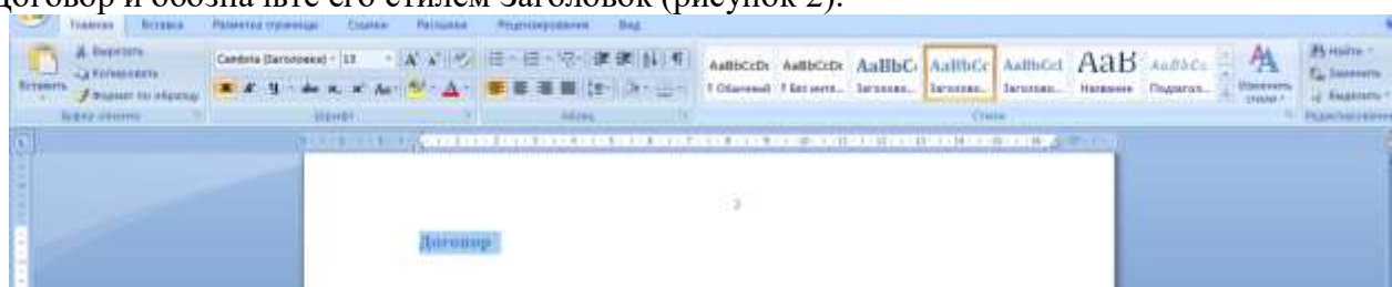
Рисунок 2. Оформление стилей
