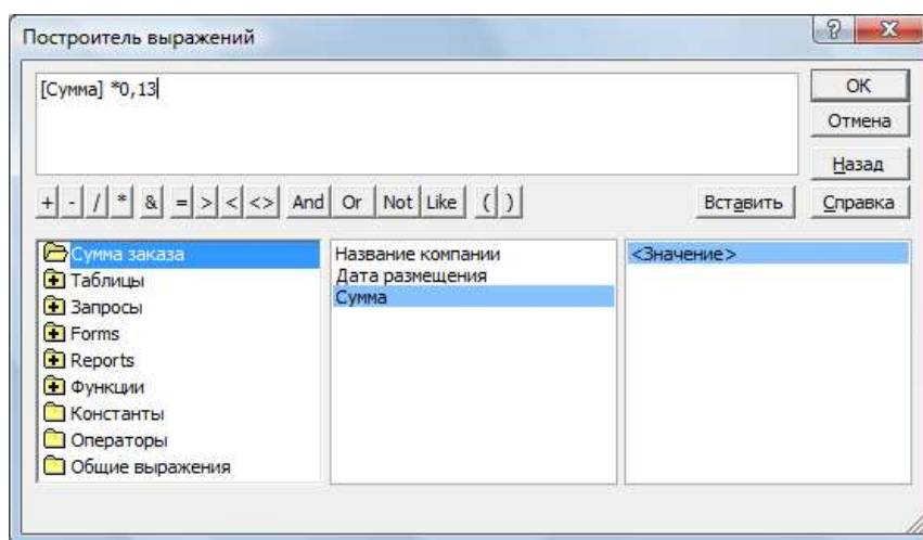
Рис. 8. Построитель выражений
