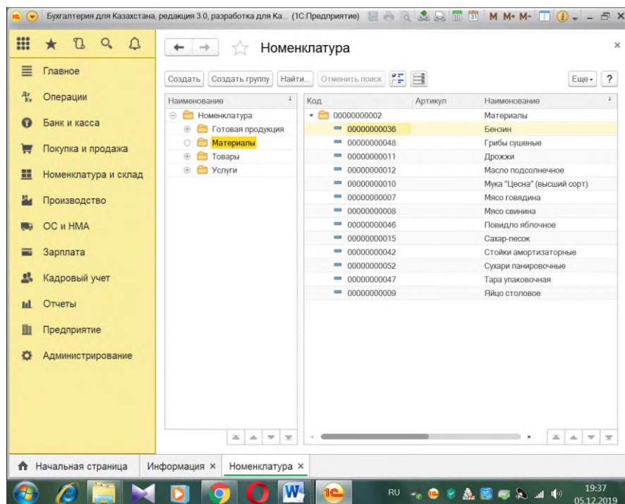
Рисунок 20 – Справочник «Номенклатура»
