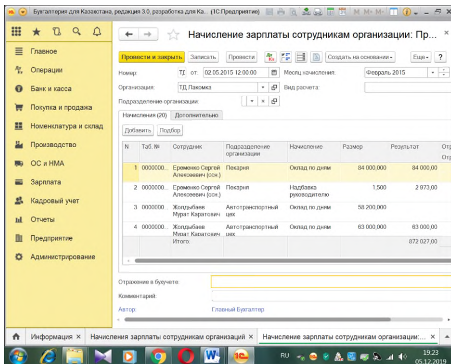
Рисунок 17 – Начисление зарплаты
