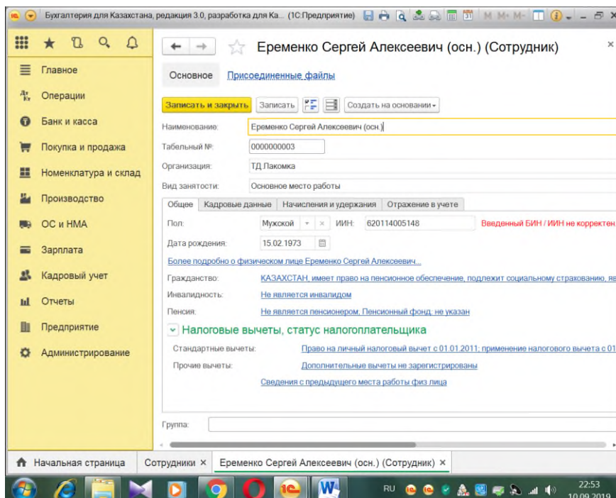
Рисунок 16 – Справочник «Сотрудники»
