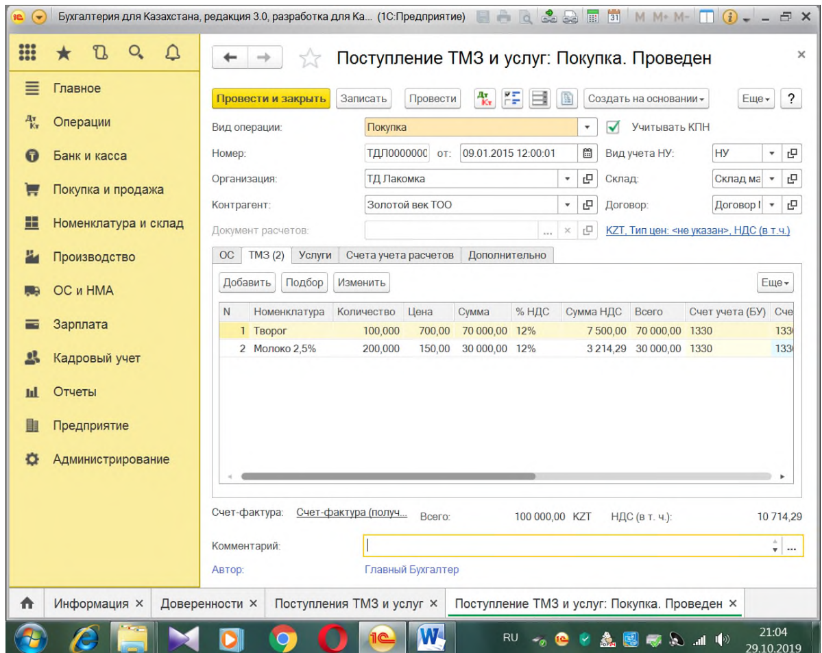
Рисунок 10 – Поступление ТМЗ
