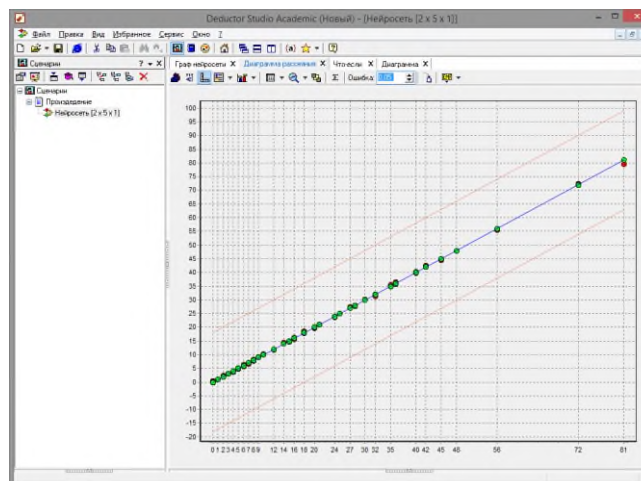
Рис. 3.9 - Диаграмма рассеяния
