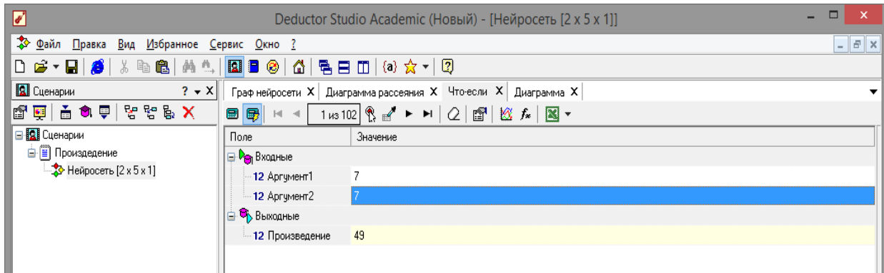
Рис. 3.11 - Инструмент «Что-Если»
