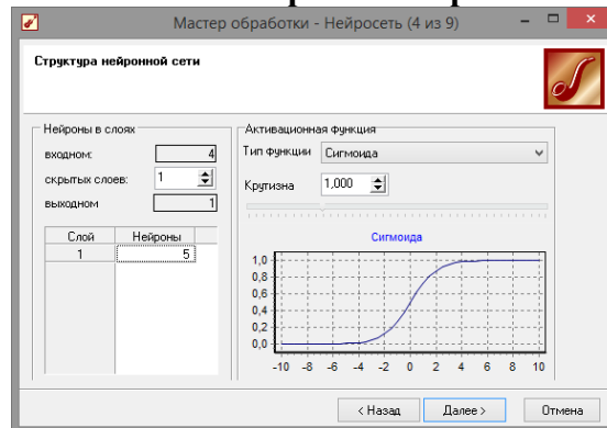
Рис. 3.20 - Настройки нейросети
