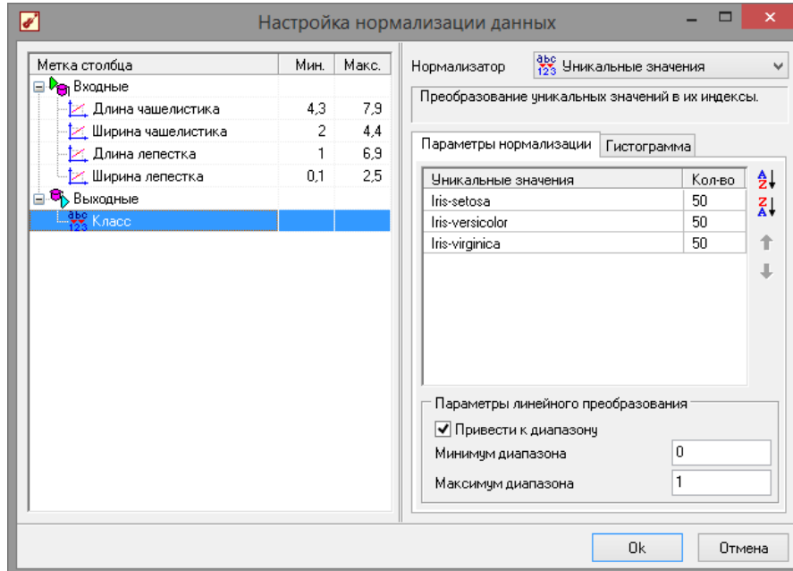
Рис. 2.13 - Настройка нормализации
