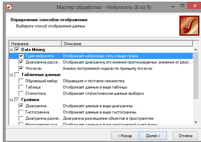
Рис. 3.7 - Обучение сети
