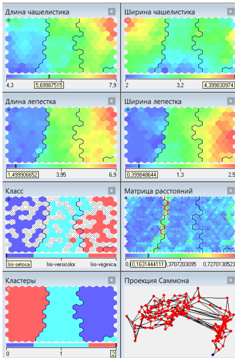
Рис. 4.11 - Карта Кохонена
