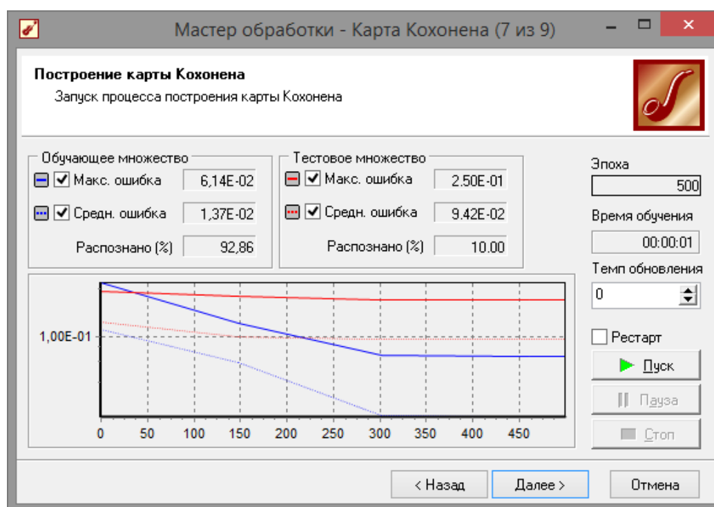
Рис. 4.8 - Процесс обучения
