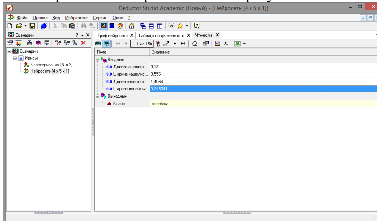
Рис. 2.22 - Инструмент «Что-Если»
