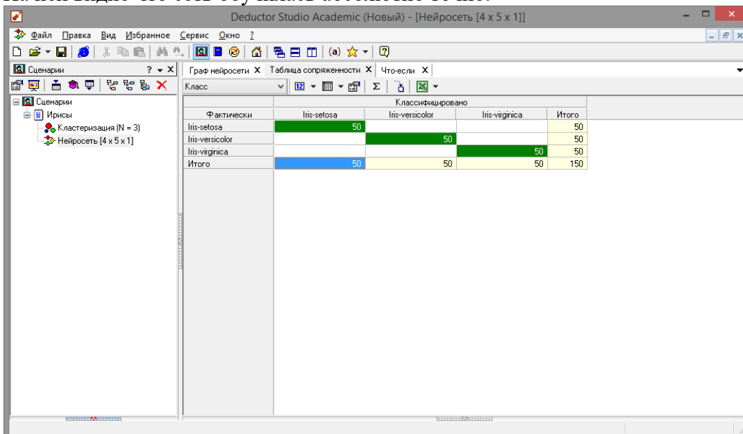
Рис. 2.21 - Диаграмма сопряженности
