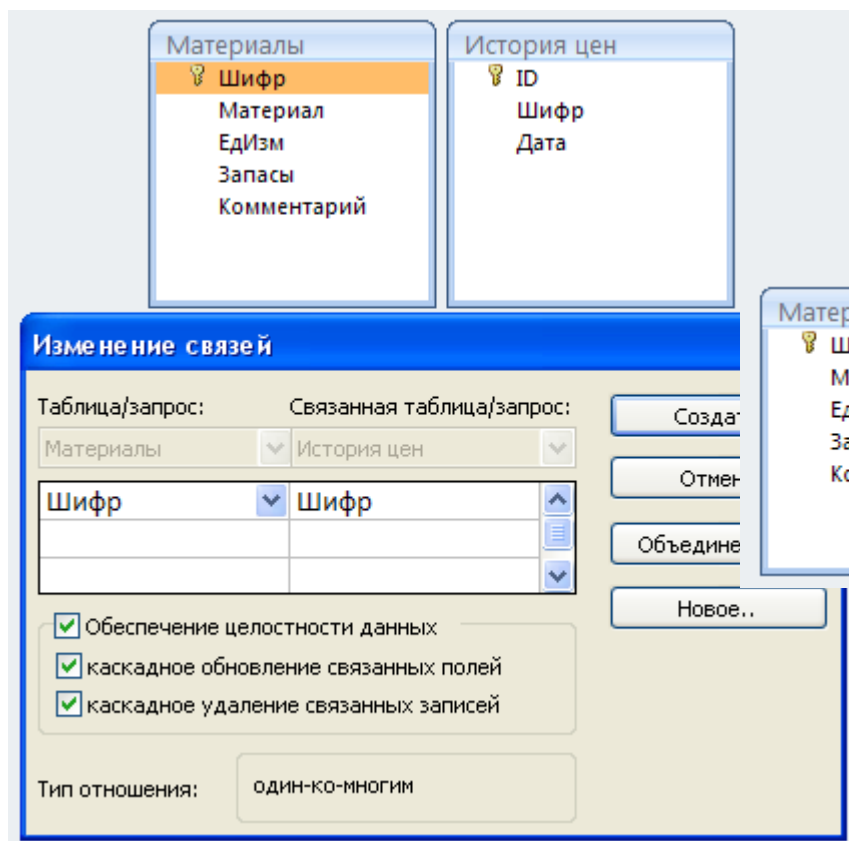
Рис. 2.3. Схема связывания полей таблиц
