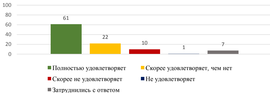
Рис. 4 Качество расписания
